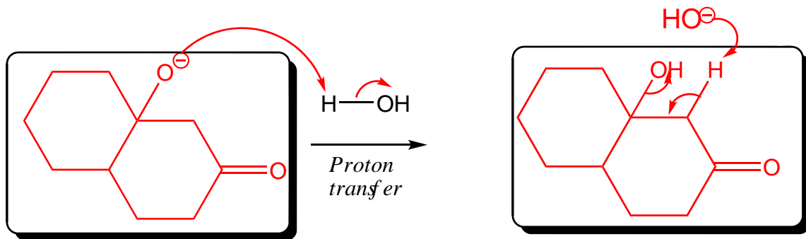
\beta -alkoxy-ketone
