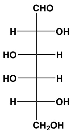
D-galactose
