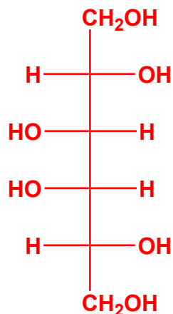
Galactitol meso; optically inactive
