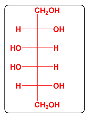
Galactitol meso; optically inactive
